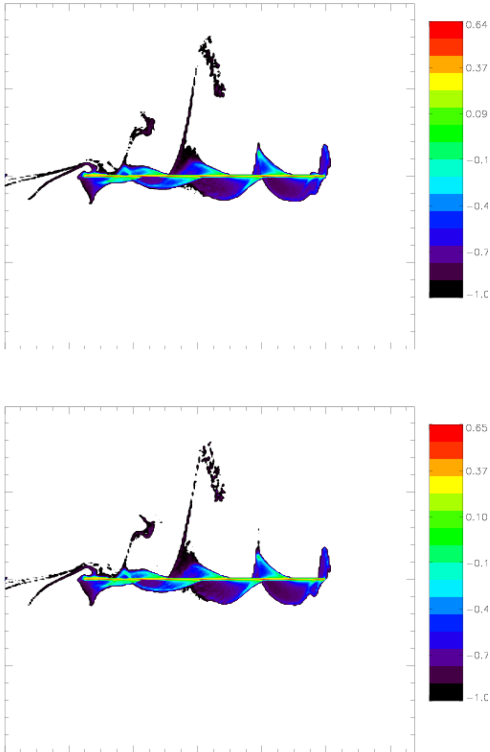
Abbildung 5.20: Teilchendichte über Impuls x und Ort x für 1 \cdot 10^{19} \text{W/cm}^2 mit Laser in y -Richtung polarisiert (oben). Darunter dieselbe Verteilung aufgetragen für eine Polarisation des Lasers in z -Richtung.
