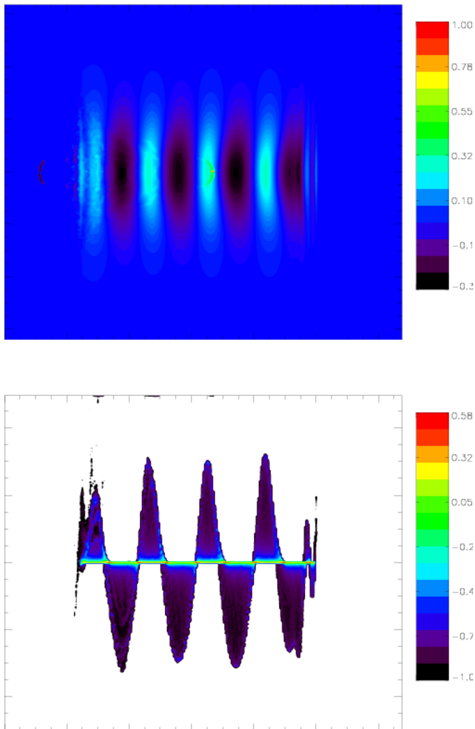
Abbildung 5.12: x -Komponente des gemittelten Impulses und Teilchendichte über Impuls x und Ort x aufgetragen (Simulation mit 2 \cdot 10^{18} \text{W/cm}^2 )
