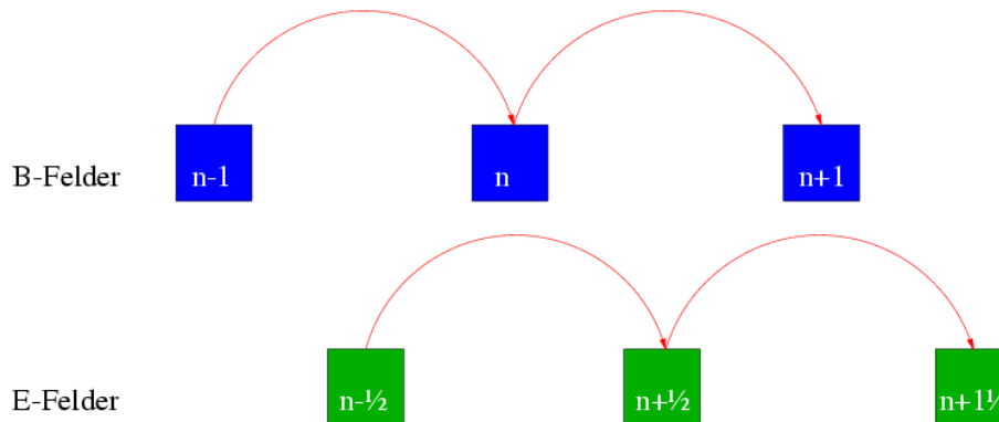
Abbildung 4.5: Der Leapfrog-Algorithmus des Maxwell-Solvers
