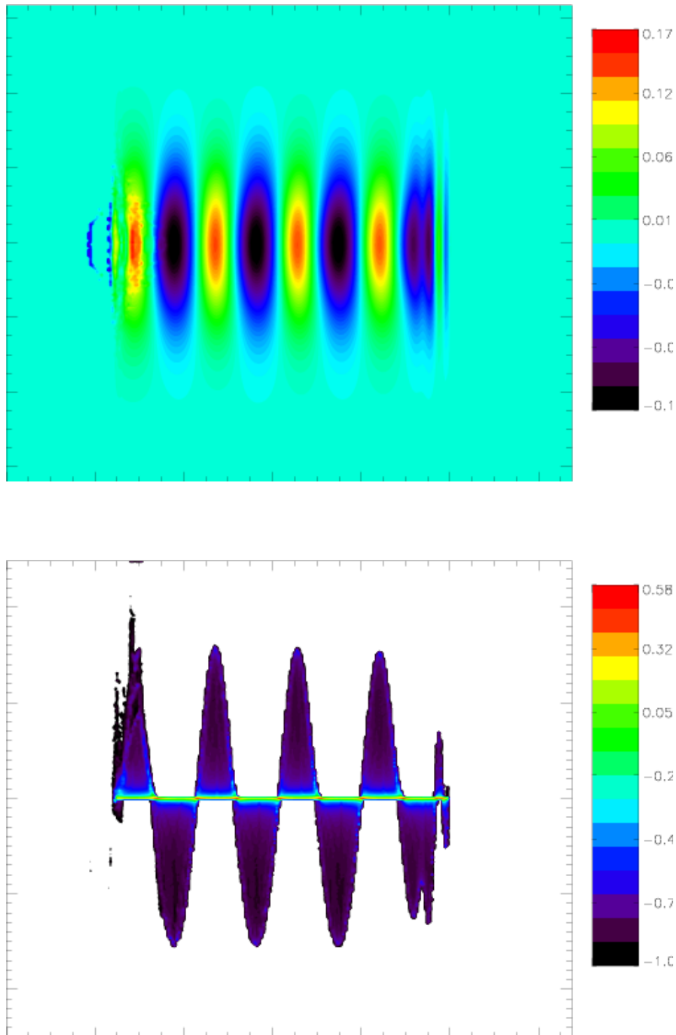
Abbildung 5.9: x -Komponente des gemittelten Elektronenimpulses und Teilchendichte gegen Impuls in x -Richtung sowie Ort x aufgetragen (Simulation mit 1 \cdot 10^{18} \text{W/cm}^2 )
