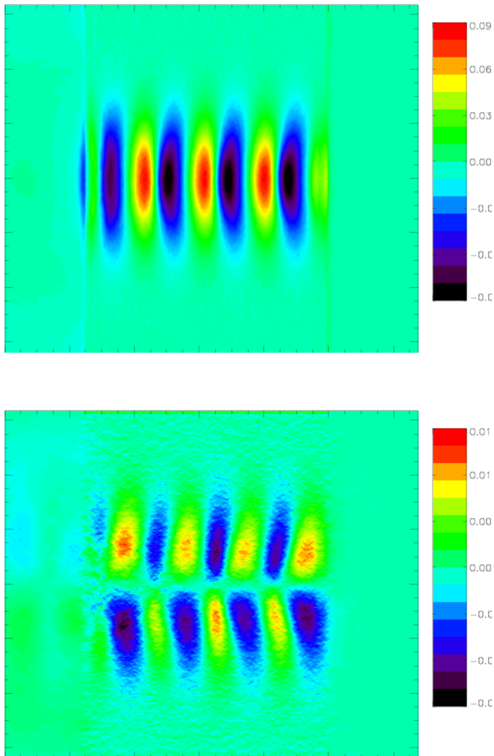
Abbildung 5.14: x - und y -Komponente der elektrischen Feldstärke einer Simulation mit 2 \cdot 10^{18} \text{W/cm}^2 und 1 \text{keV}
