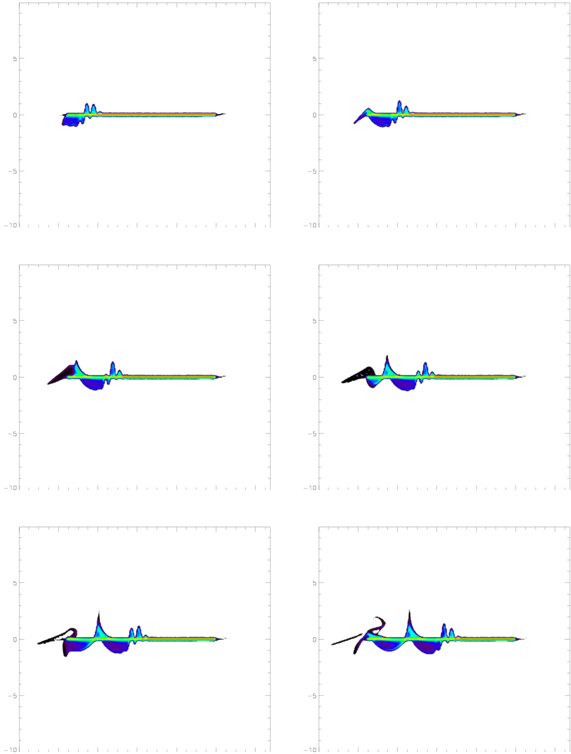
Abbildung 5.17: Verschiedene Phasen der Entstehung schneller Teilchen an der Grenzfläche und im Inneren des Plasmas bei 1 \cdot 10^{19} \text{W/cm}^2 und einer Plasmatemperatur von 1 keV.
