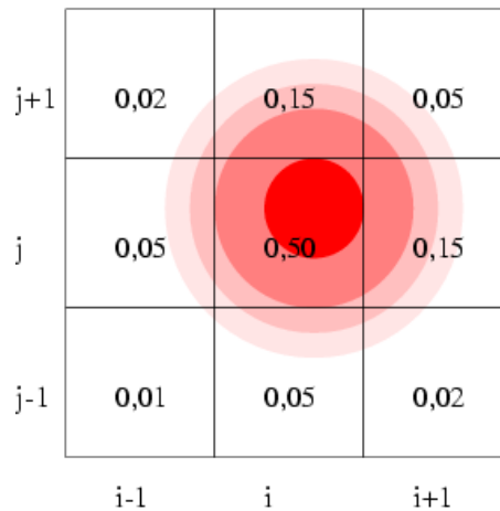
Abbildung 4.3: Gewichtung höherer Ordnung
