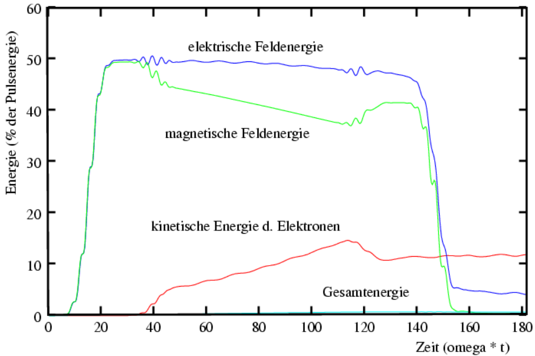
Abbildung 5.6: Energiebilanz einer Simulationen mit 5 \cdot 10^{18} \text{W/cm}^2
