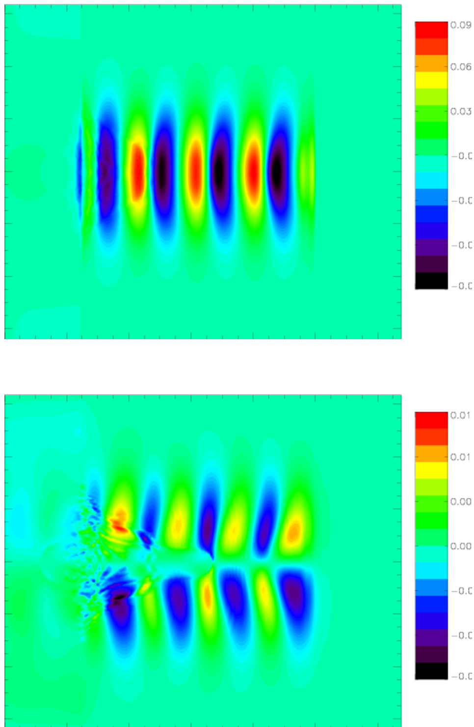
Abbildung 5.11: x - und y -Komponente der elektrischen Feldstärke einer Simulation mit 2 \cdot 10^{18} \text{W/cm}^2
