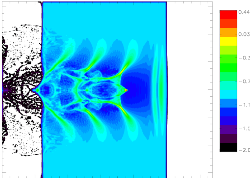
Abbildung 5.15: Elektronendichte normiert auf n_{crit} einer Simulation mit 2 \cdot 10^{19} \text{W/cm}^2
