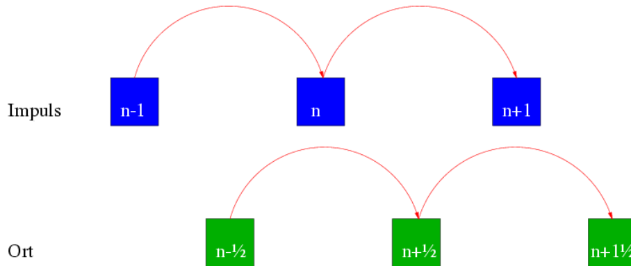
Abbildung 4.6: Der Leapfrog-Algorithmus des Teilchenmovers
