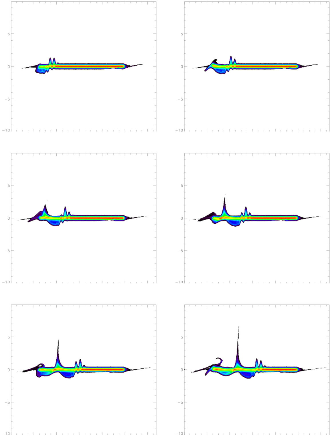
Abbildung 5.18: Verschiedene Phasen der Entstehung schneller Teilchen an der Grenzfläche und in Inneren des Plasmas bei 1 \cdot 10^{19} \text{W/cm}^2 und einer Plasmatemperatur von 10 keV.
