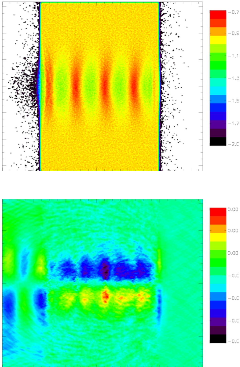
Abbildung 5.13: Elektronendichte und z -Komponente der magnetischen Feldstärke einer Simulation mit 2 \cdot 10^{18} \text{W/cm}^2 und 1keV
