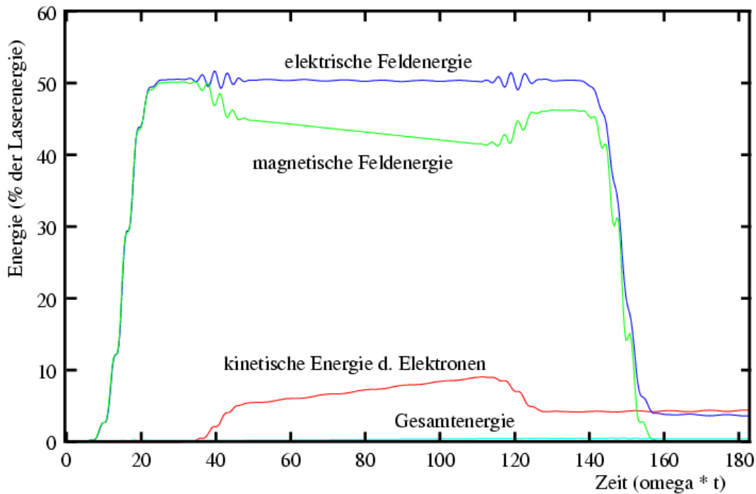
Abbildung 5.5: Energiebilanz einer Simulationen mit 2 \cdot 10^{18} \text{W/cm}^2
