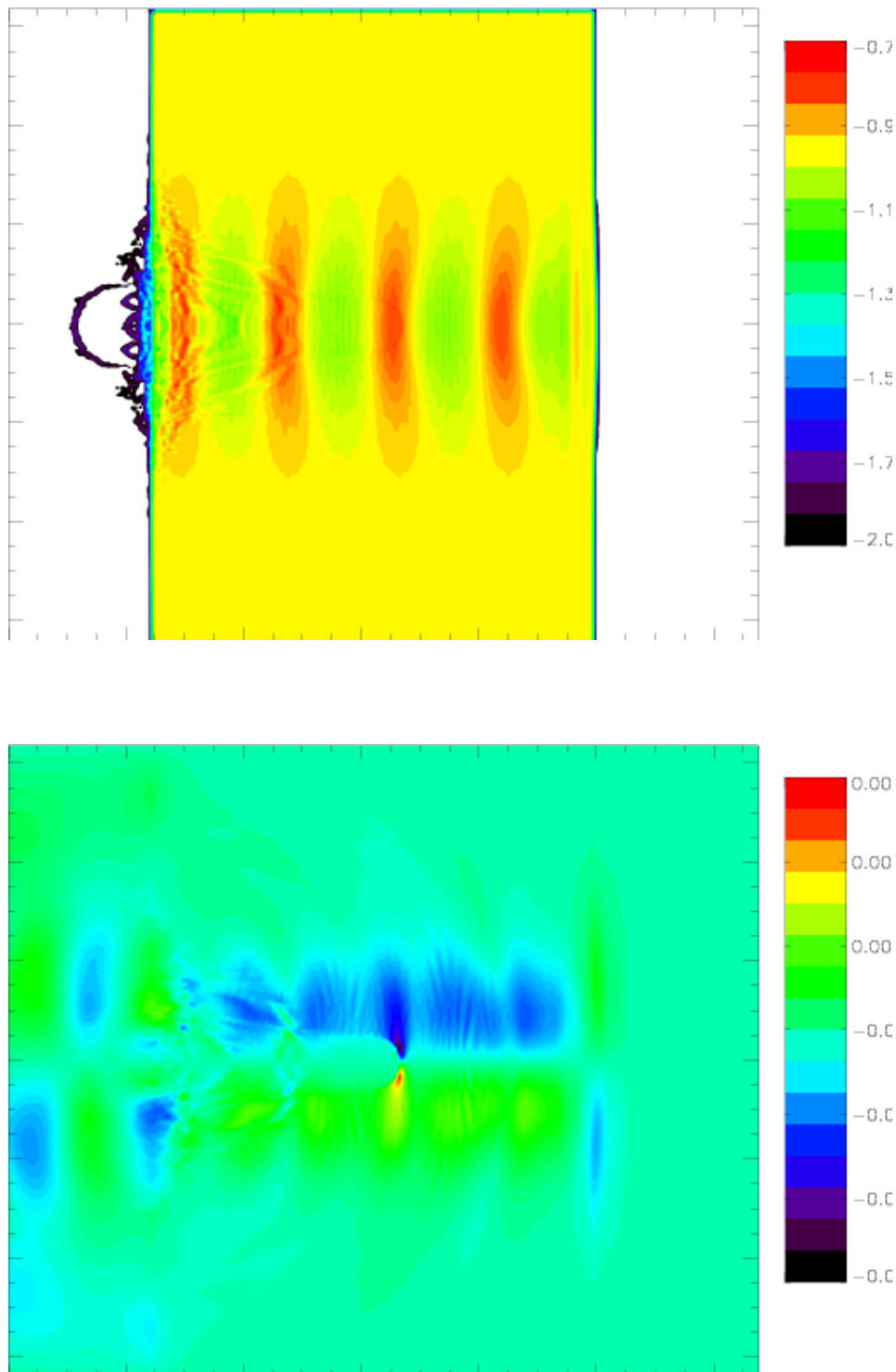
Abbildung 5.10: Elektronendichte und z -Komponente der magnetischen Feldstärke einer Simulation mit 2 \cdot 10^{18} \text{W/cm}^2
