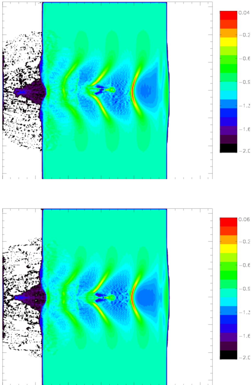
Abbildung 5.19: Teilchendichte über Ort x und y für 1 \cdot 10^{19} \text{W/cm}^2 mit Laser in y -Richtung polarisiert (oben). Darunter dieselbe Verteilung aufgetragen für eine Polarisation des Lasers in z -Richtung.
