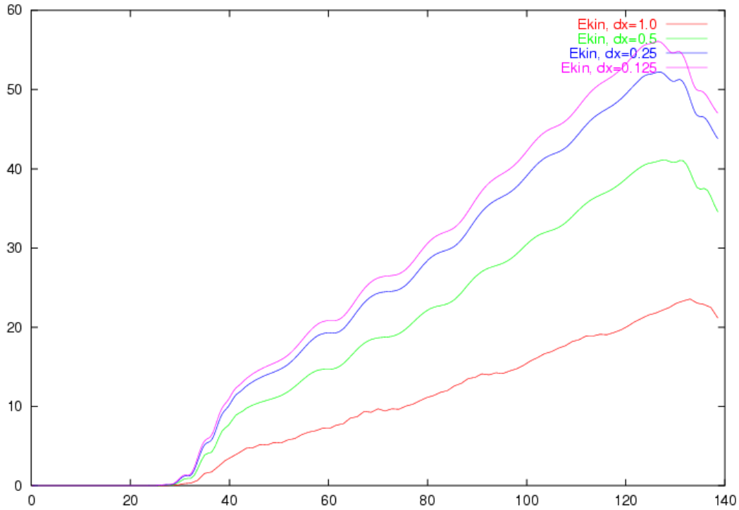
Abbildung 5.2: Bilanz der Teilchenenergie der Simulation mit verschiedenen Schrittweiten
