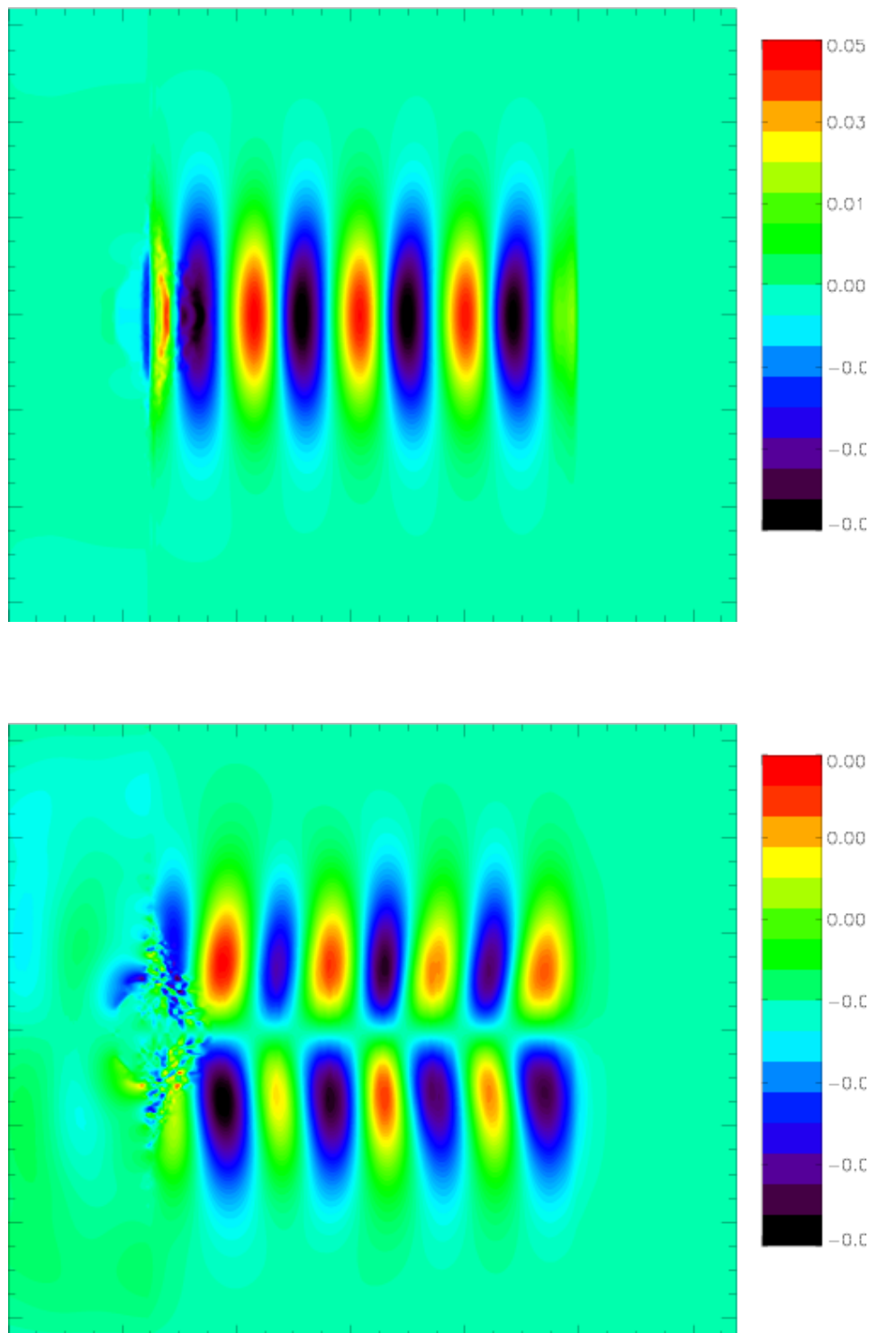
Abbildung 5.8: Elektrische Feldstärken in x - und y -Richtung der Simulation aus Abbildung 5.7 mit 1 \cdot 10^{18} \text{W}/\text{cm}^2
