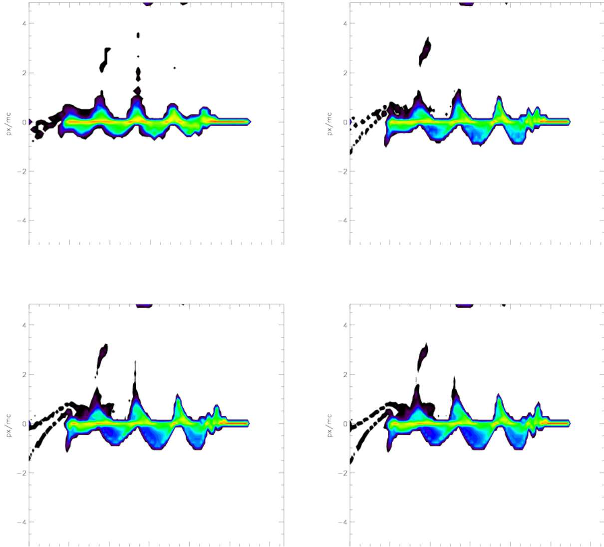
Abbildung 5.4: Elektronendichten über Impuls x / Ort x für Schrittweiten von 1.0/k (oben links) bis 0.125/k (unten rechts).
