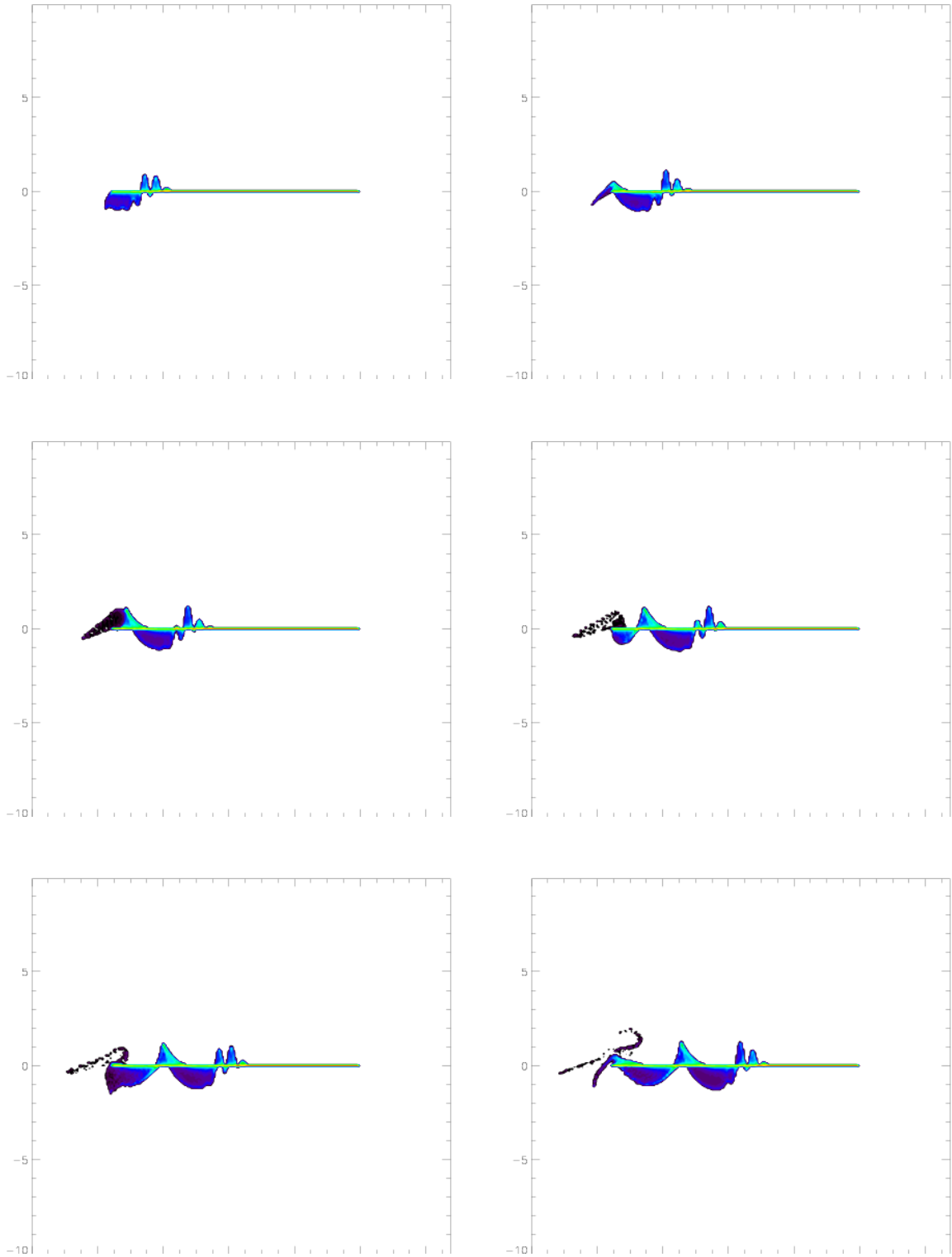
Abbildung 5.16: verschiedene Phasen der Entstehung schneller Teilchen an der Grenzfläche zwischen Vakuum und Plasma bei 1 \cdot 10^{19} \text{W/cm}^2 im Fall kalten Plasmas
