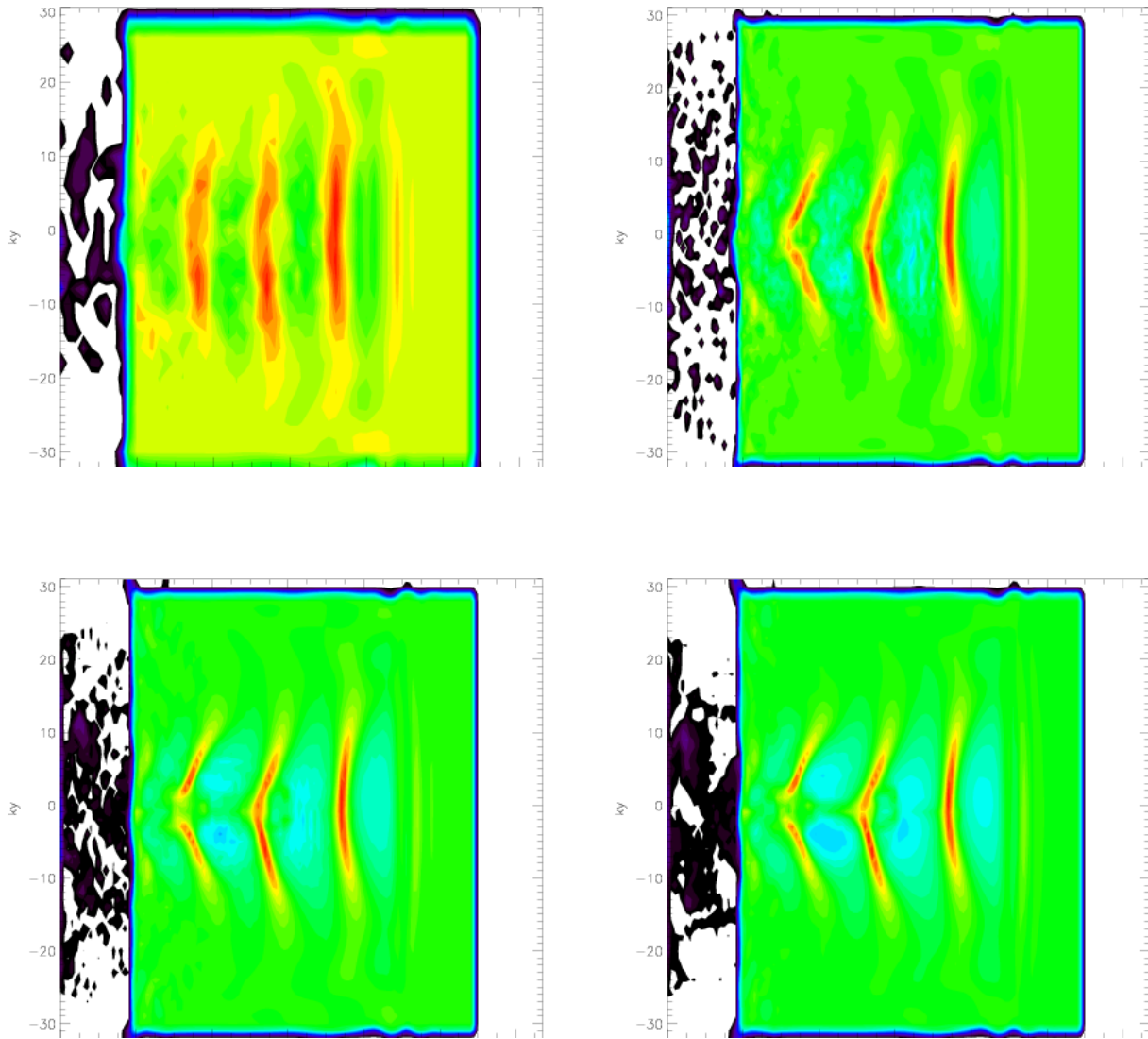
Abbildung 5.3: Elektronendichten über Ort für Schrittweiten von 1.0/k (oben links) bis 0.125/k (unten rechts).
