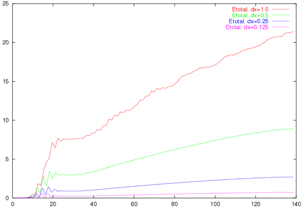
Abbildung 5.1: Gesamtenergiebilanz der Simulationen mit verschiedenen Schrittweiten
